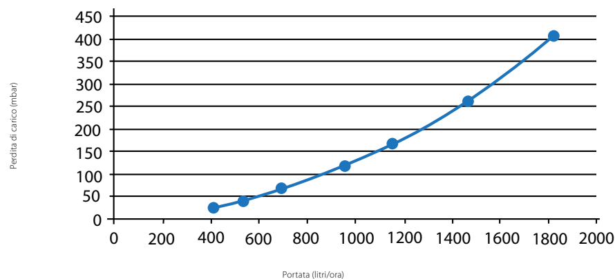
Prestige 24-32 Solo/Excellence - perdita di carico in base alla portata
