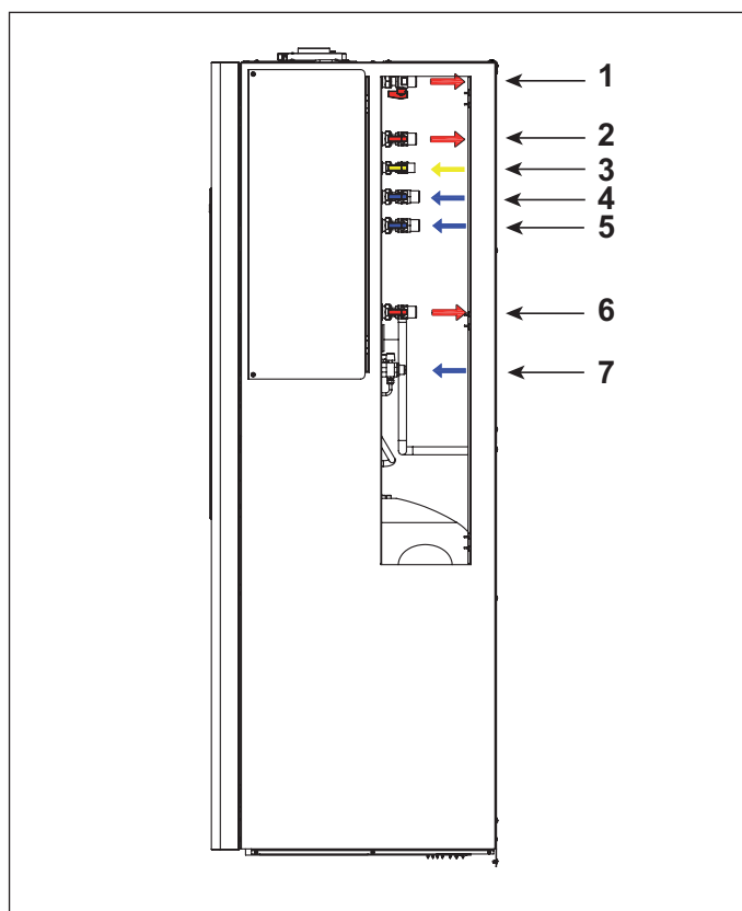
Fig. 5 Schema idraulico Giava KRB V
