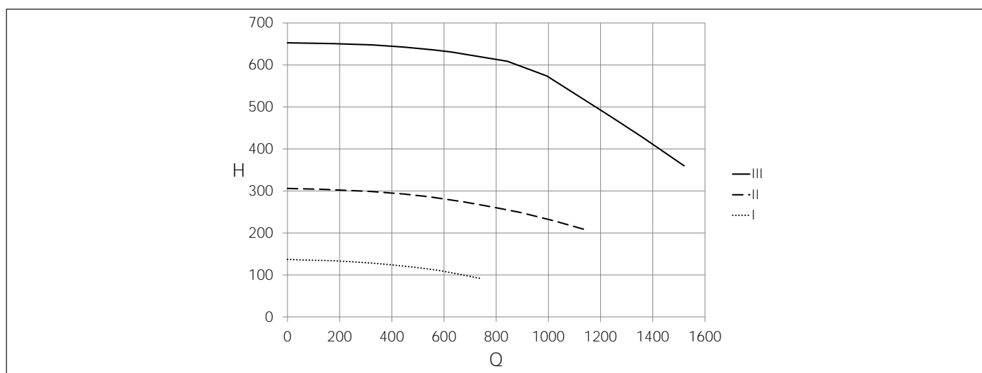
Fig. 23 Prevalenza disponibile zona bassa temperatura 1 (KRB V - KRB Z)
