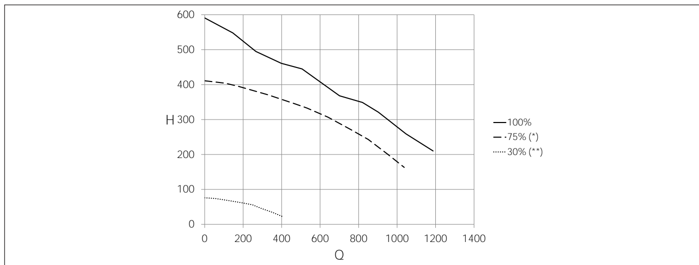
Fig. 21 Prevalenza disponibile KRB 32
