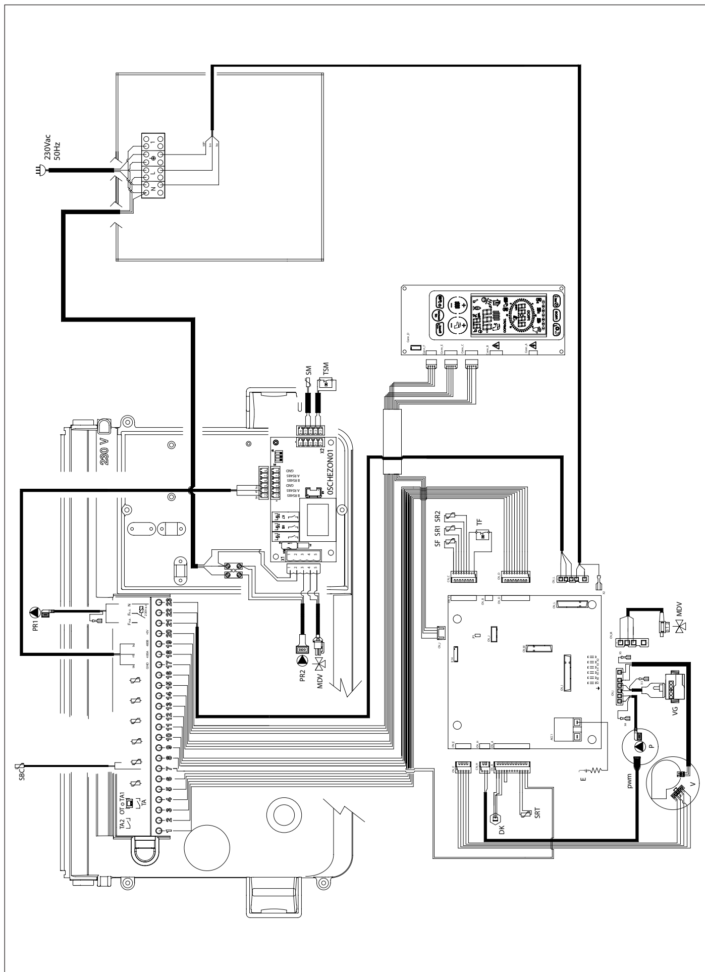
Fig. 26 Schema elettrico KRB-V
