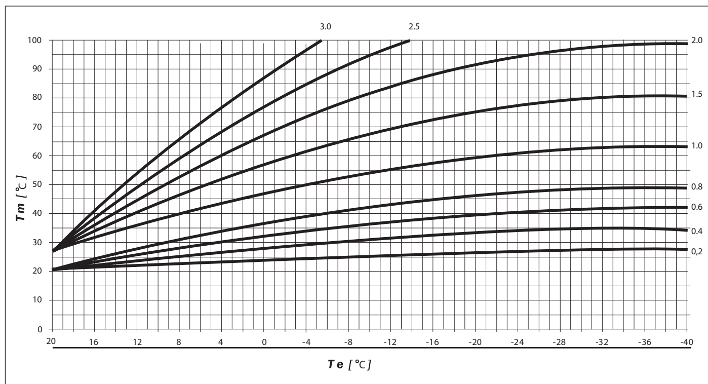
Fig. 17 Curve di termoregolazione
