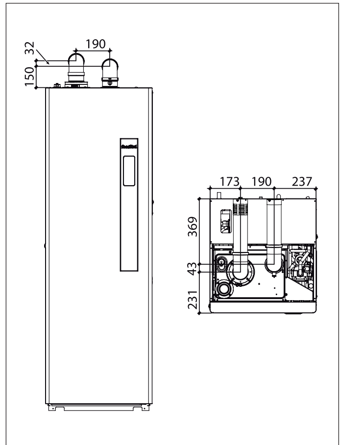
Fig. 12 Dimensioni condotti coassiali tipo C43 - C53 - C83
