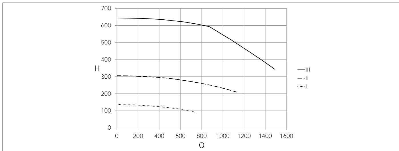
Fig. 24 Prevalenza disponibile zona bassa temperatura 2 (KRB Z)
