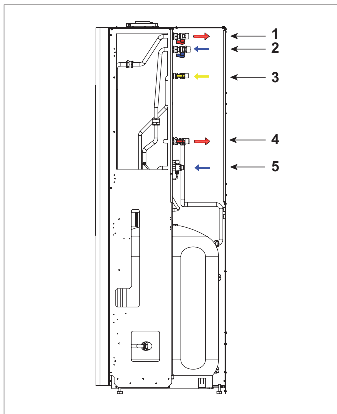
Fig. 4 Schema idraulico Giava KRB
