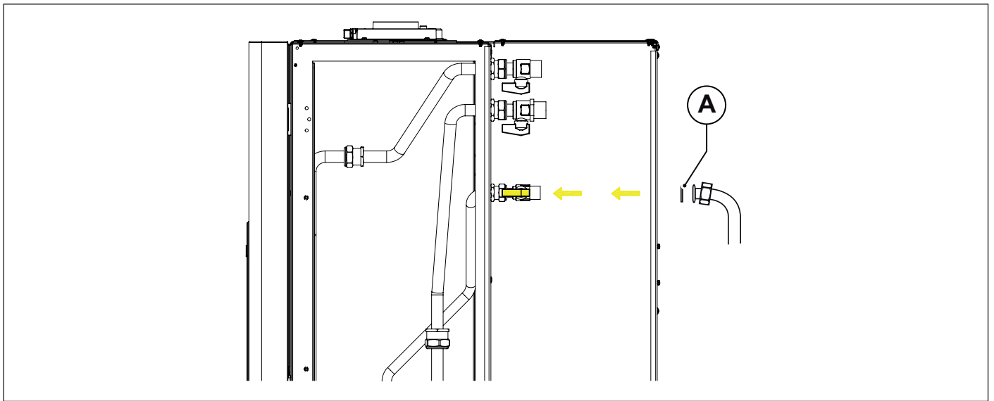
Fig. 15 Allacciamento alla rete del gas
