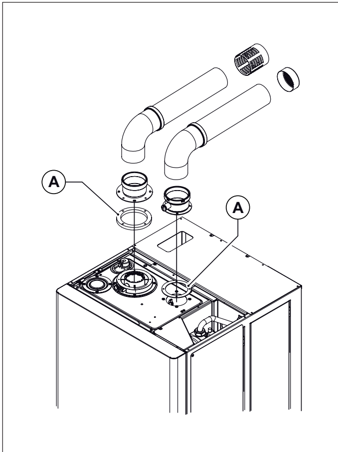
Fig. 11 Condotti coassiali tipo C43 - C53 - C83
