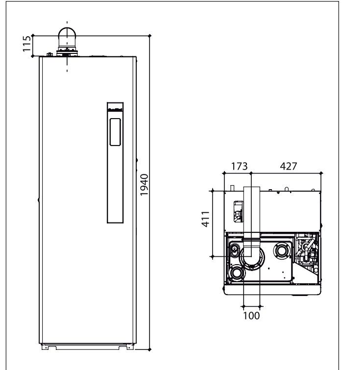
Fig. 10 Dimensioni condotti coassiali tipo C33
