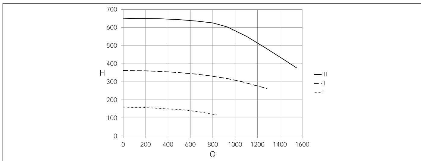
Fig. 22 Prevalenza disponibile zona alta temperatura (KRB V - KRB Z)
