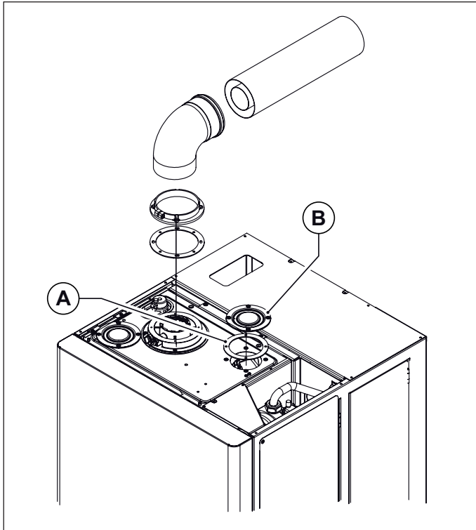
Fig. 9 Condotti coassiali tipo C33
