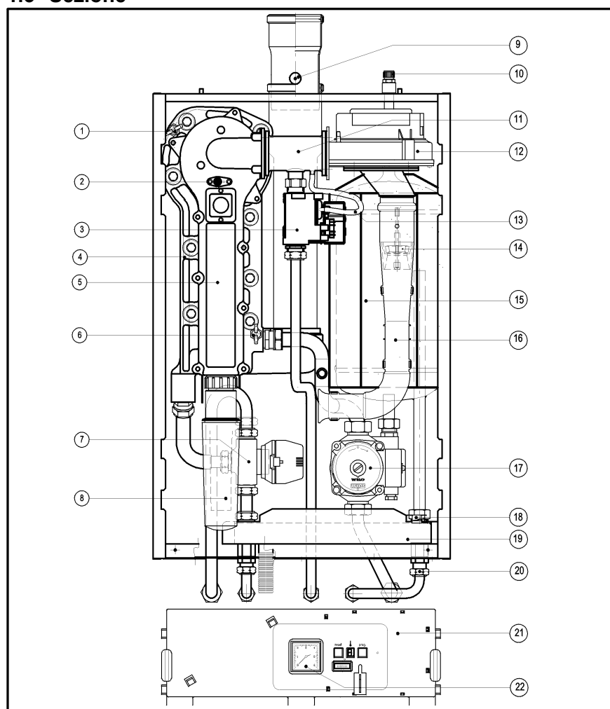
Fig. 1: sezione
