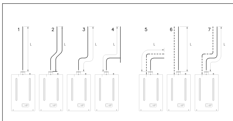
Fig. 8: sistema di scarico coassiale
