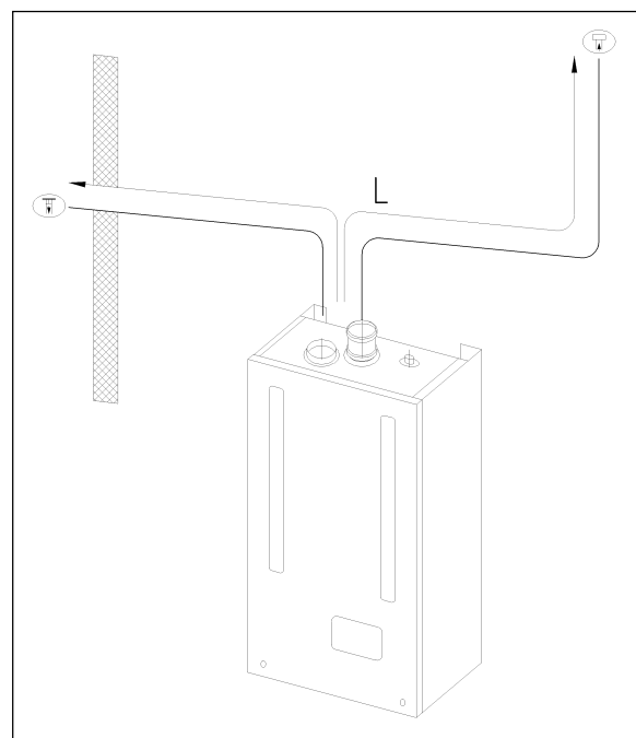
Fig. 10: sistema di scarico parallelo
