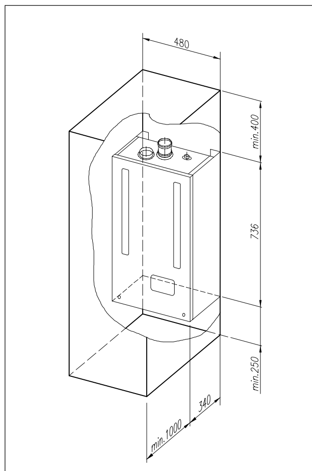
Fig. 7: ingombro
