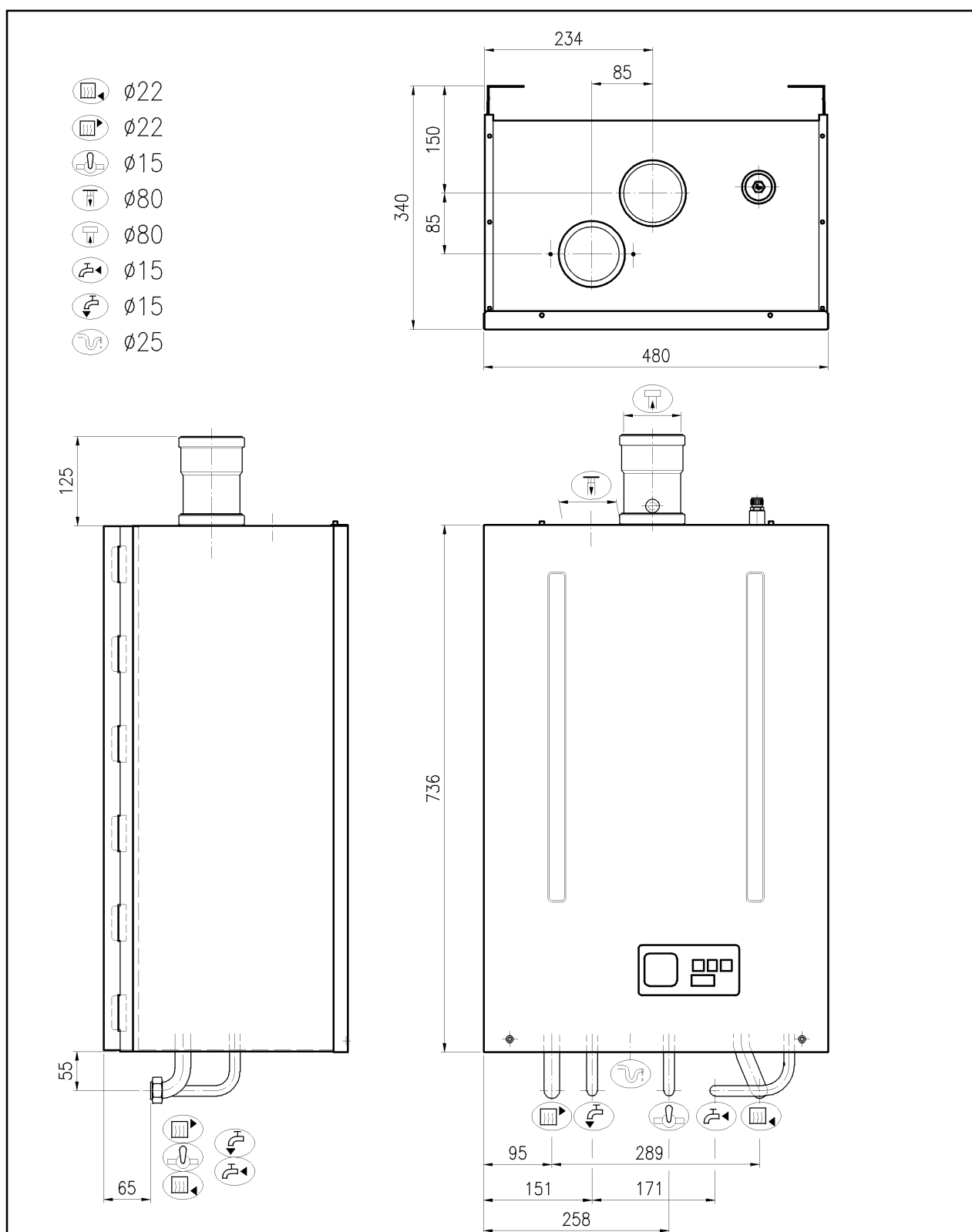
Fig. 2: dimensioni
