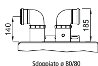
Sdoppiato ø 80/80
